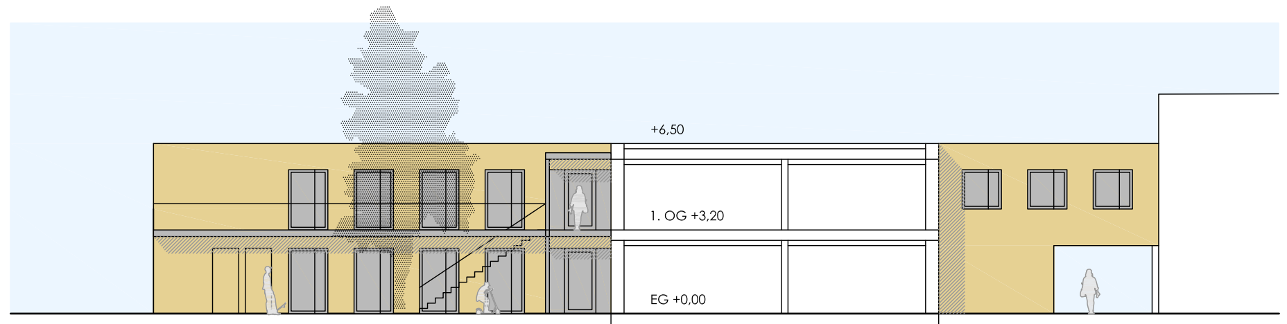
SCHNITT / ANSICHT OST
