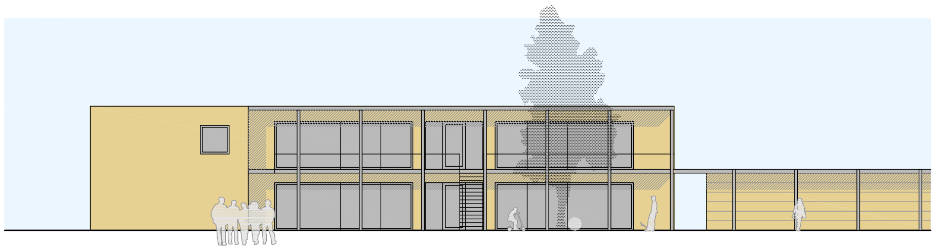
ANSICHT SÜD
